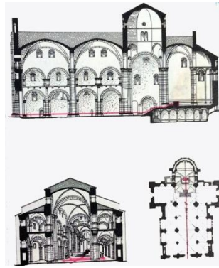
Basilica Romanica, sezioni e pianta
